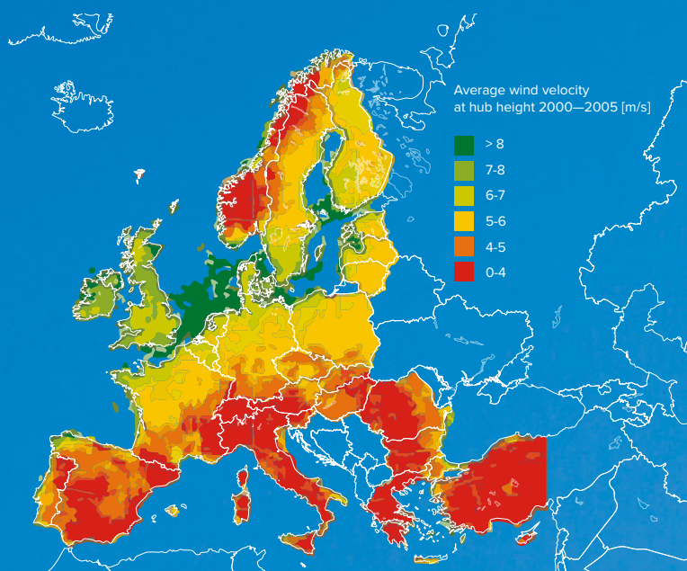
Gemiddelde windsnelheden in Europa
